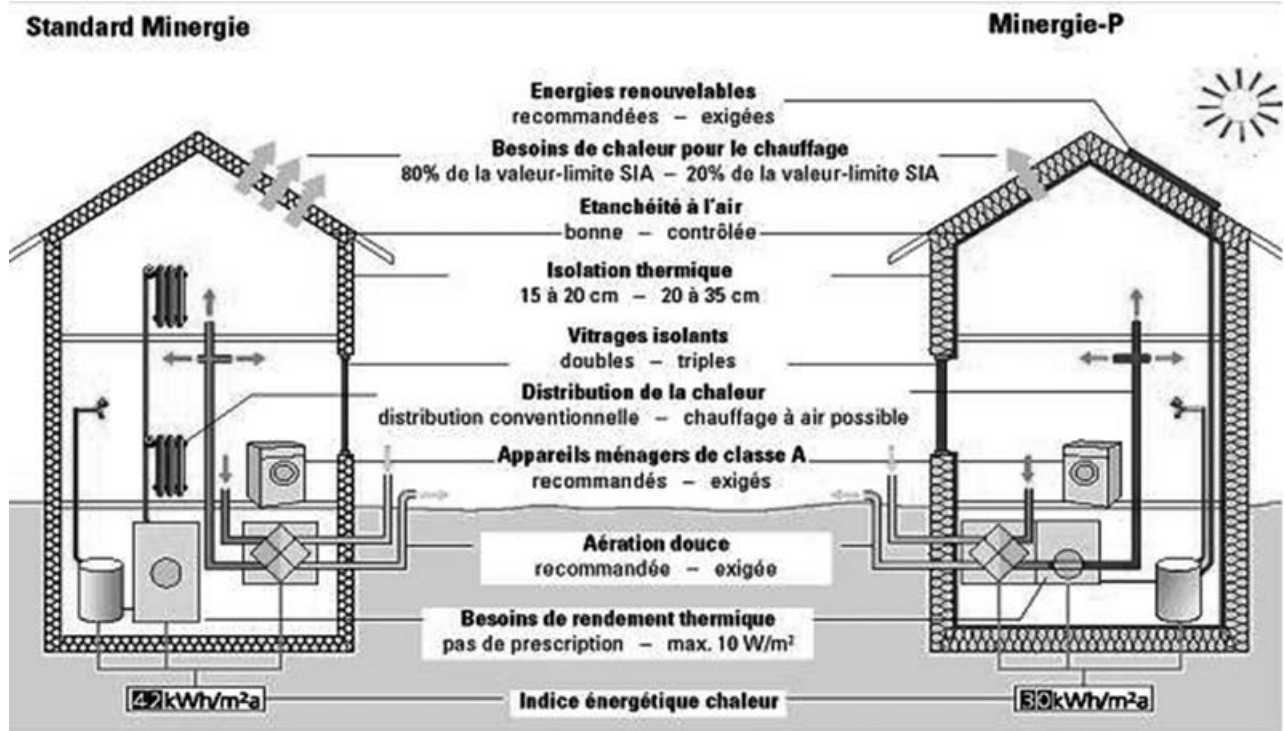
Caractéristiques d'un immeuble Minergie® et d'un immeuble Passivhaus (dénommé en Suisse Minergie-P®)
